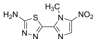
Megazol
