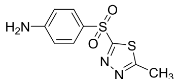
Sulfamethizole
