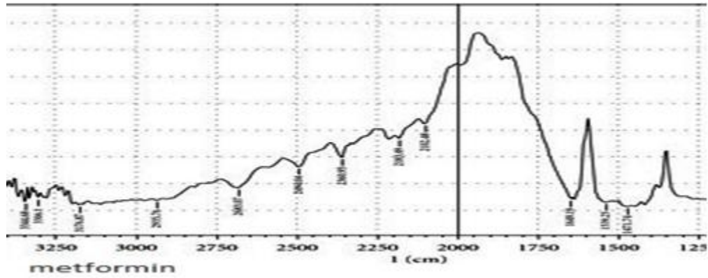
Fig. 1.FTIR of metformin
