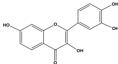
Fisetin
