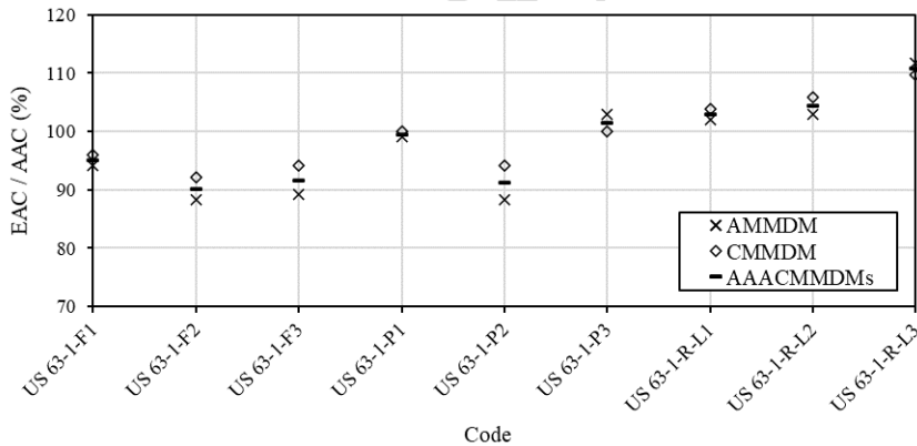
Fig. 12. EAC per AAC values for the US 63-1 mixes
