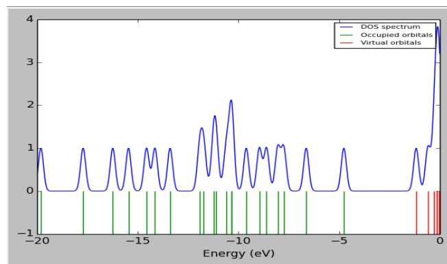
DFT/6-311+G (d)
