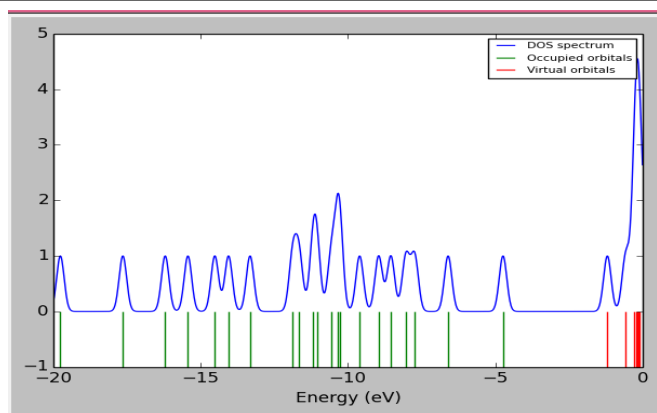
DFT/6-31++G (d, p)
