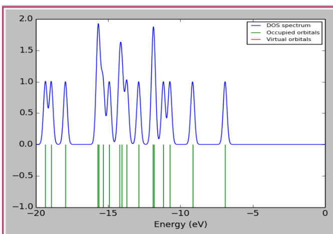
RHF/6-311+G (d)
