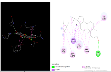
c) Kaempferol- 10.2
