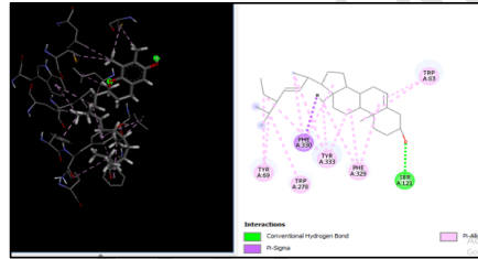
b) Tocopherol – 8.1
