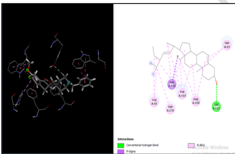
e) Donepezil-10.9
