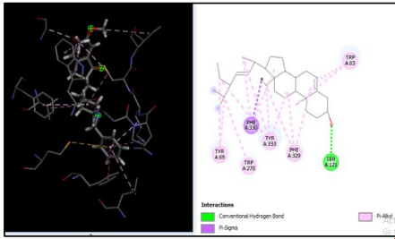
e) Donepezil-8.8
