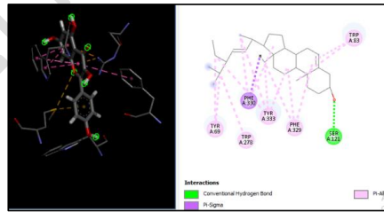
b) Kaempferol- 8.5
