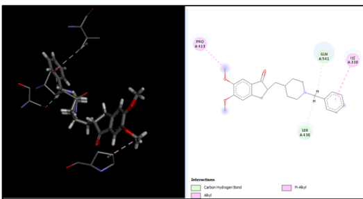
e) Donepezil -7.6
