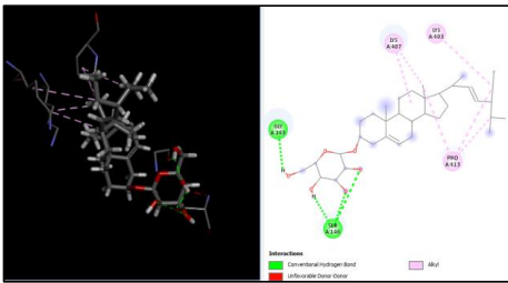
c) Stigmasterol -6.4
