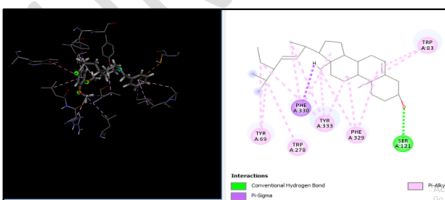
e) Donepezil- 8.7
