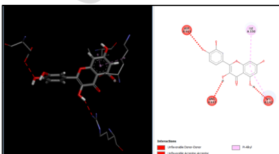
a) Quercetin -7.3
