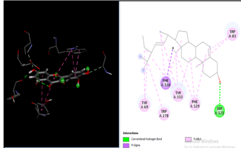
b) Quercetin – 10.4
