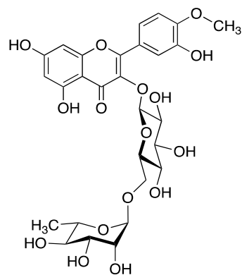
Isorhamnetin-3-O-rutinoside (3)
