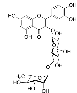
Rutin (1)
