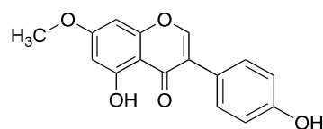
Prunetin (2)
