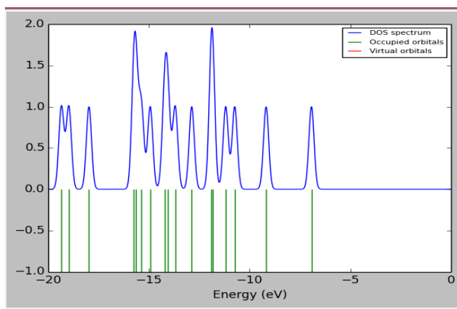
RHF/6-31++G (d, p)
