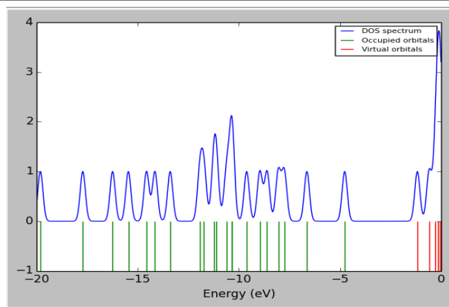
DFT/6-311+G (d)
