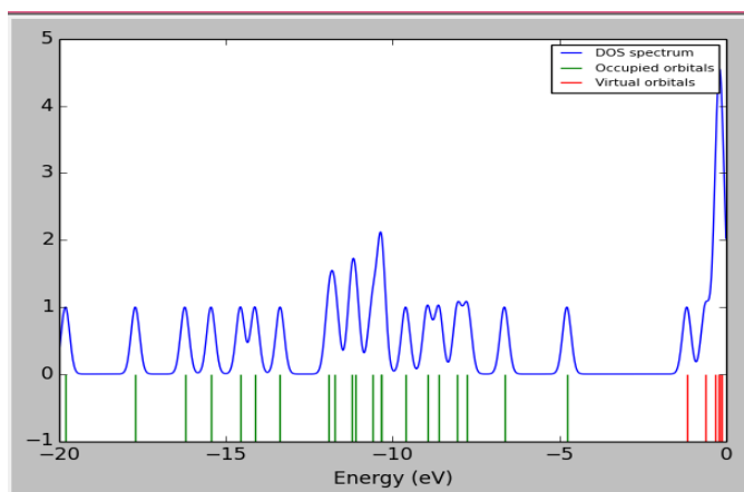
DFT/6-311++G (d, p)
