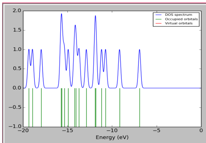
RHF/6-311+G (d)
