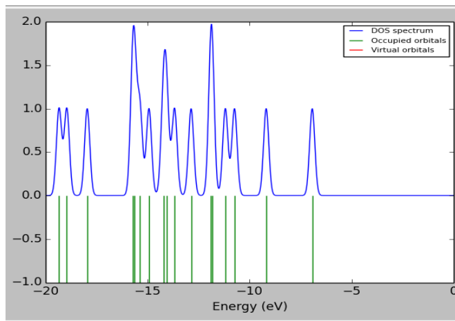
RHF/6-311++G (d, p)
