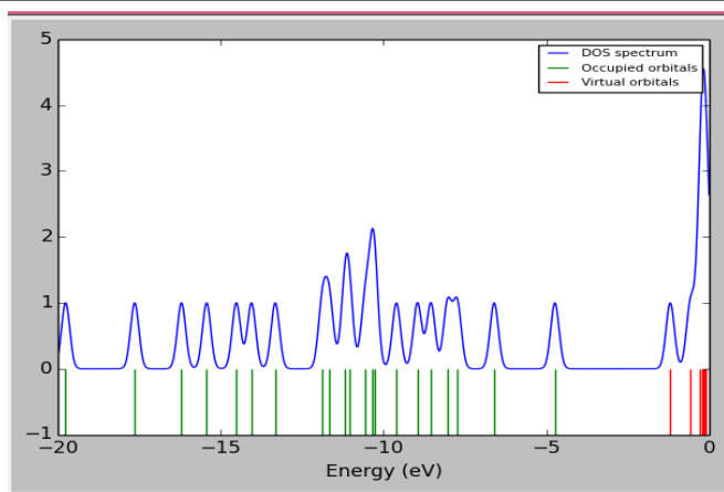
DFT/6-31++G (d, p)
