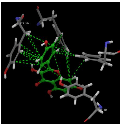
B) Kaempferol -10.39
