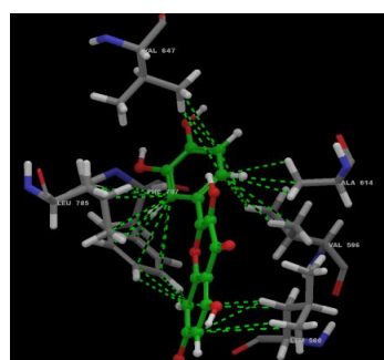
B) Quercetin -11.72
