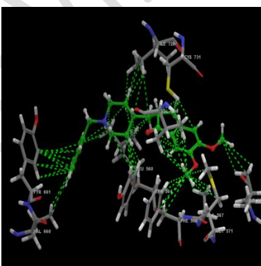
F) Donepezil -6.63
