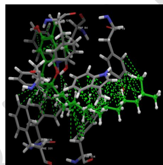
E) Tocopherol -8.76
