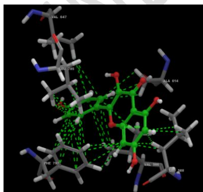
A) Kaempferol -12.23
