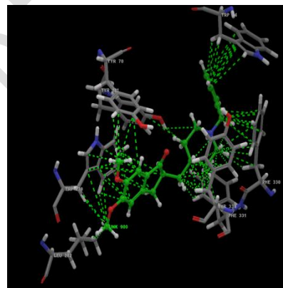
F) Donepezil -11.98
