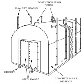
Fig. 5 Missouri type charcoal kiln[36]
