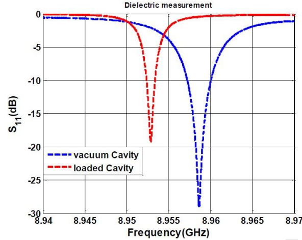
Fig. 3. Frequency-dependent reflection parameter
