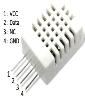
Fig. 2. DHT22
