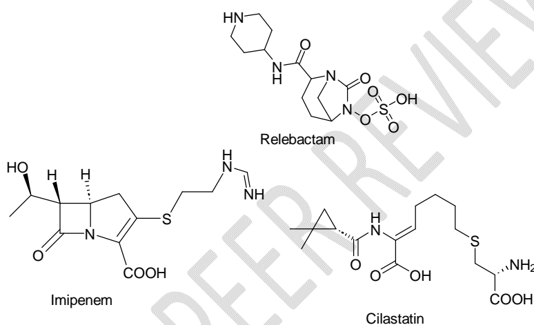
Figure 20 : Association imipénem-cilastatine-relebactam
