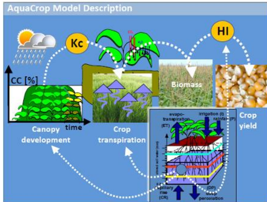
Fig 1 : AquaCropModel
