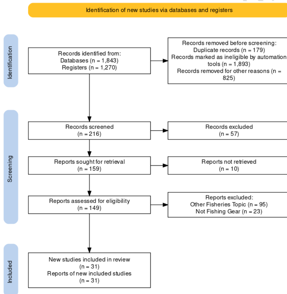
Fig. 1. Prisma Diagram
