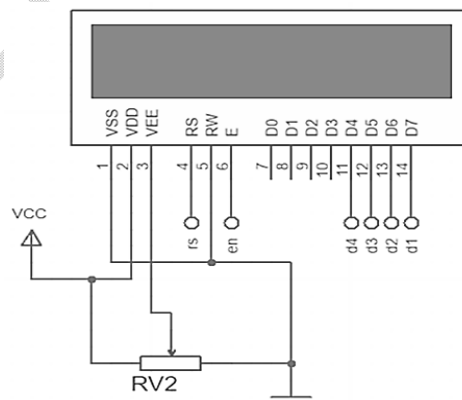
Fig. 4 LCD1 LMO16L Unit
