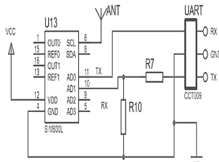
Fig. 5 SIM 800L unit
