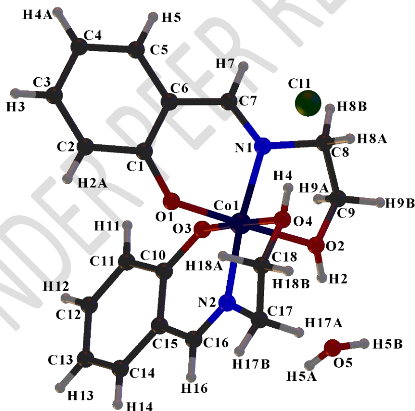
Fig. 1. Crystal structure of the complex [Co(HL) 2 ].Cl·H 2 O
