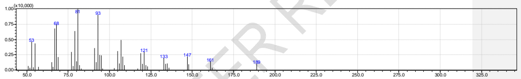
Elemene <beta->
