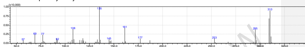
Avobenzene
