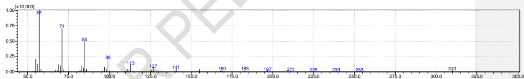
Docosane <n->
