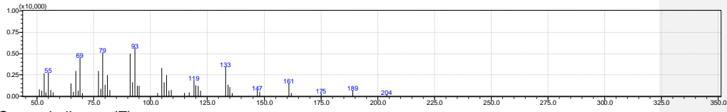
Caryophyllene <Z>
