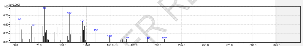
Javanol
