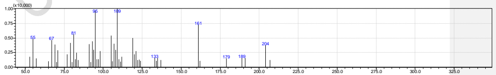
Copaborneol
