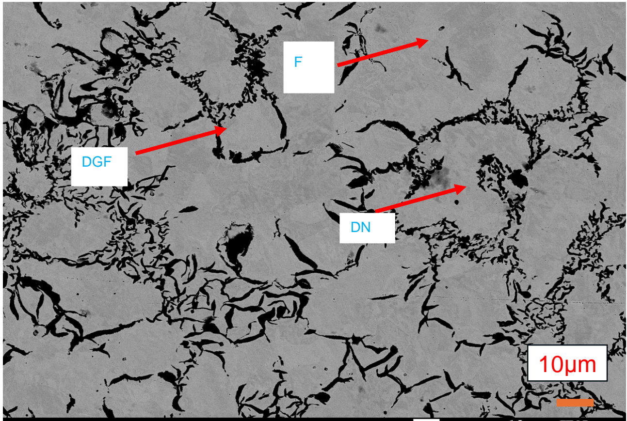
Figure 5: A5 SEM image
