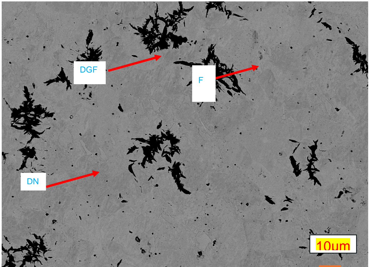
Figure 3: A3 SEM image
