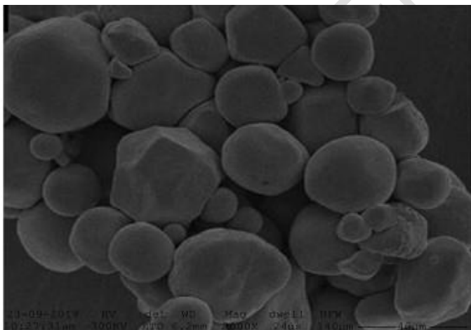
Fig 16: SEM of sample A3
