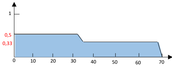
Fig. 4 Agrégation des sorties des règles selon Zadeh
