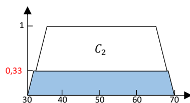
Fig. 2 : Coupure de la sortie 2
