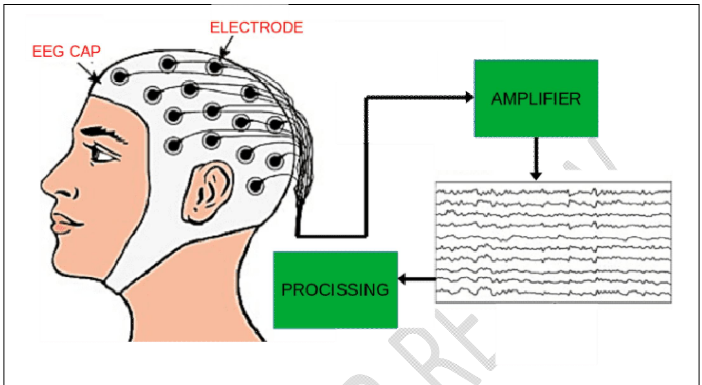
Figure.1. EEGrecordingssystem[5].
