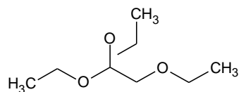
Ethoxyacetaldehyde diethylacetal CCOC(OC)OC
