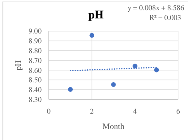
2.1 pH
