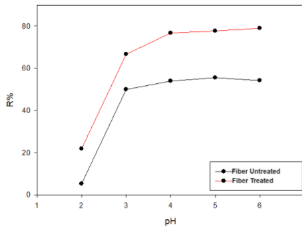
Figura 06: Influencia do pH na adsorção do níquel por fibras de sisal.
