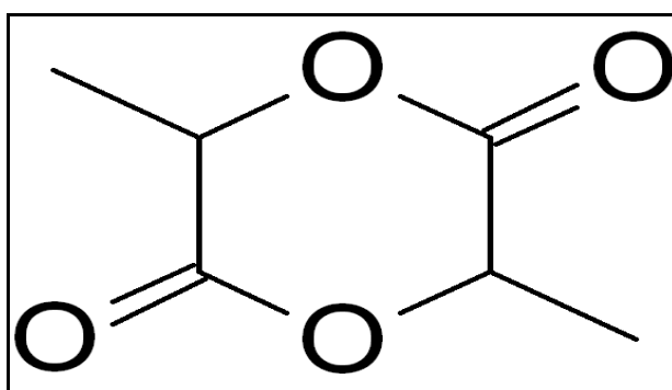
Fig No 4: - Lactide [2]
