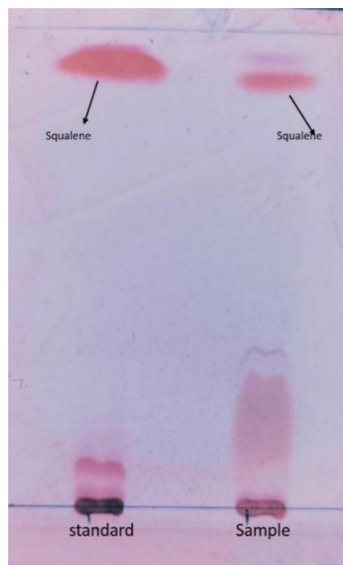
Figure 1: TLC squalene
