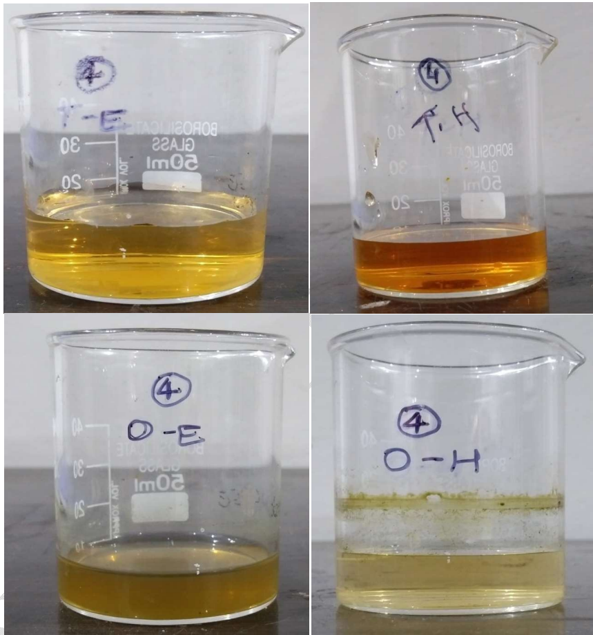
Fig.12: Testfortannins
