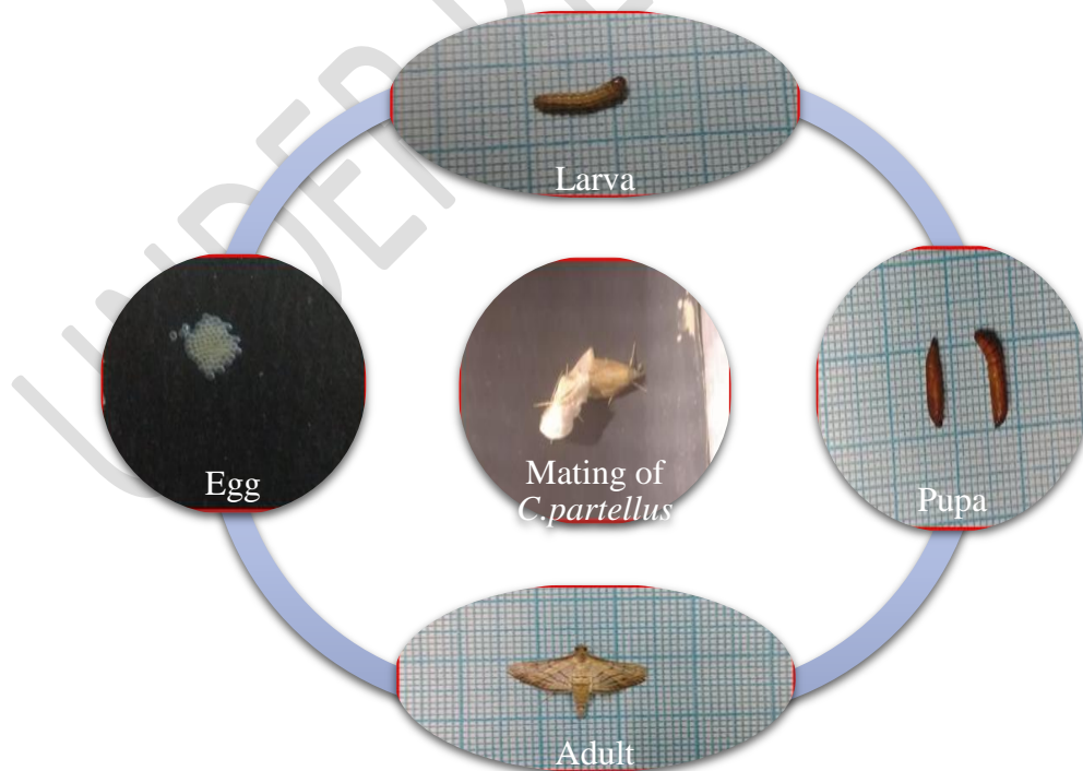
Fig 1. Life Circle of Chilopartellus .
