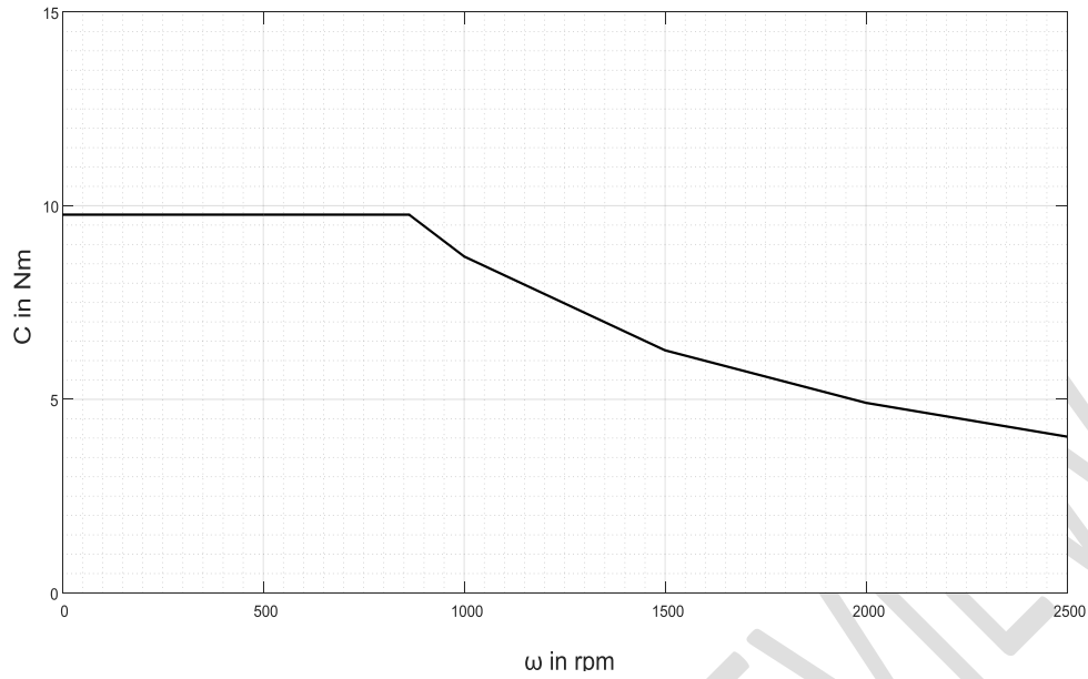
Fig.9- Cωlimitingcurve: AcetalDuracon M90.
