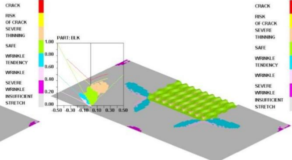
(b2) S=1.0\text{mm}/W=1.0\text{mm}
