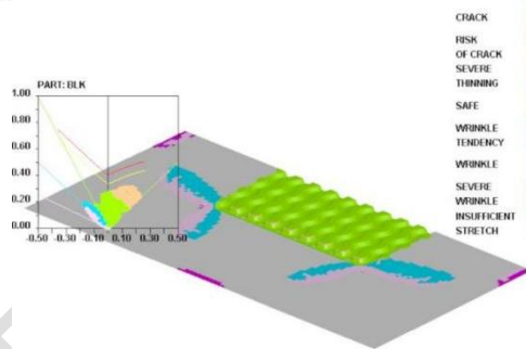
(b3) S=1.0\text{mm}/W=1.5\text{mm}
