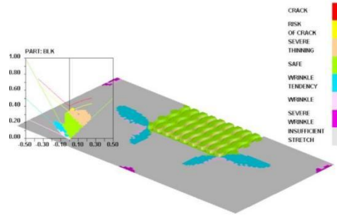
(a3) S=0.5\text{mm}/W=1.5\text{mm}
