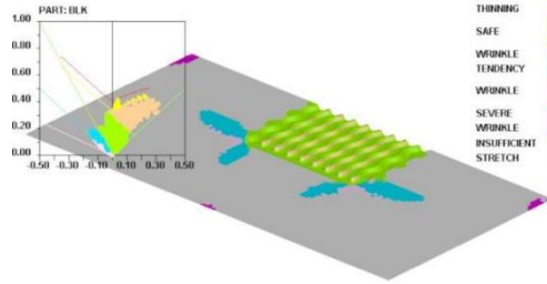
(b1) S=1.0\text{mm}/W=0.75\text{mm}
