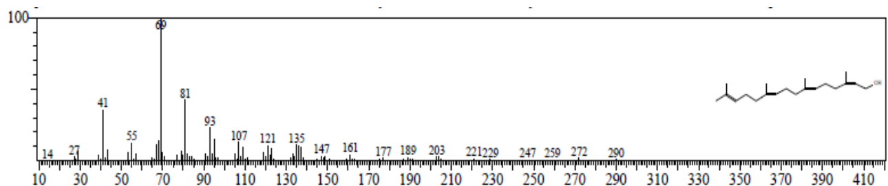
Fig. 13. Mass spectrum of Hexadeca-2,6,10,14-tetraen-1-ol, 3,7,11,16-tetramethyl- (RT: 31.054, Area % = 1.34)
