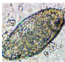
Plate 3 S. intercalatum
