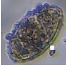
Plate1 F. hepatica
