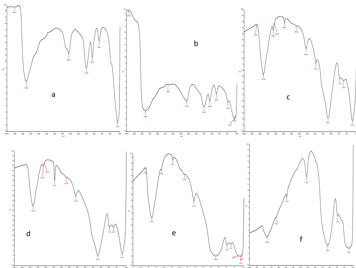
Fig. 5: The FTIR Spectrum of (a) JF (b) JA (c) JCI (d) JC2 (e) MN (f) CN
