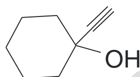
1-ethynyl-1-cyclohexanol
