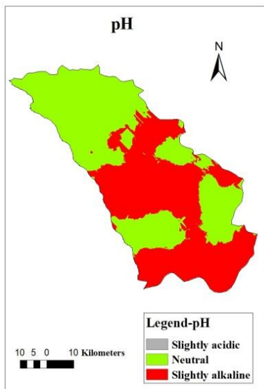
Fig. 13. Ordinary kriging
