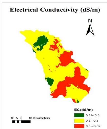
Fig. 17. Ordinary kriging
