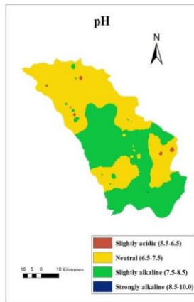
Fig. 14. IDW
