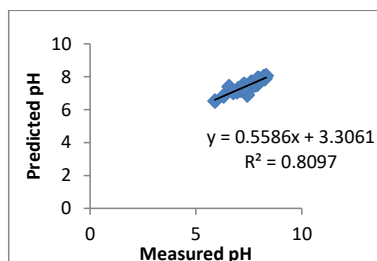
Fig. 21. Soil pH
