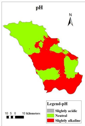
Fig. 13. Ordinary kriging
