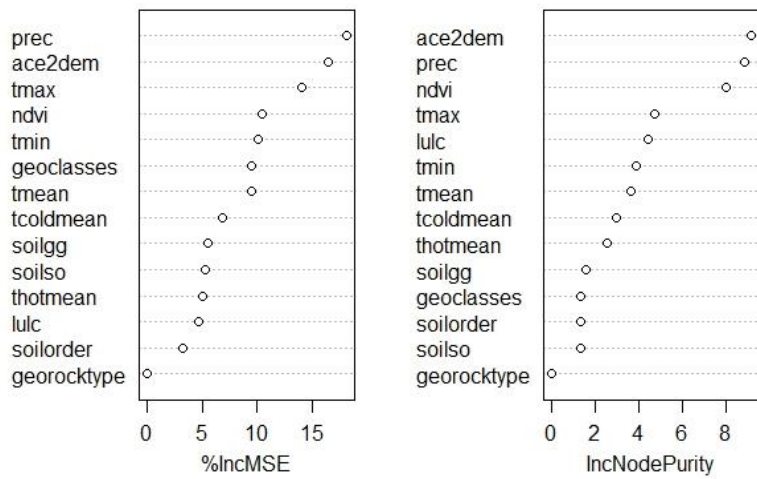
Fig. 11. Soil pH
