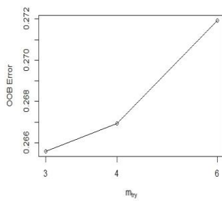
Fig. 9. Soil pH
