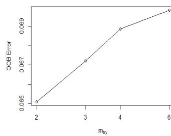
Fig. 10. EC
