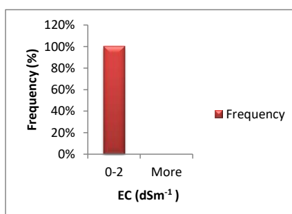
Fig. 6. EC (dSm -1 )
