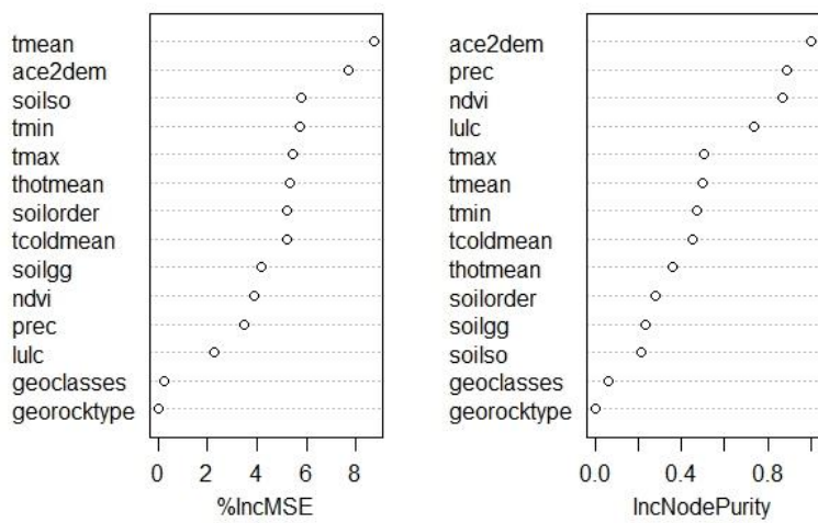
Fig. 12. EC
