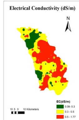
Fig. 18. IDW
