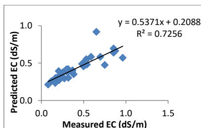
Fig. 22. EC (dS/m)
