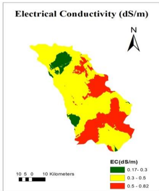
Fig. 17. Ordinary kriging
