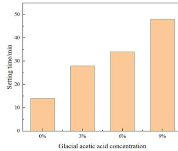
Fig.3Effectofglacialaceticacidconcentrationonsolidificationtime [26]
