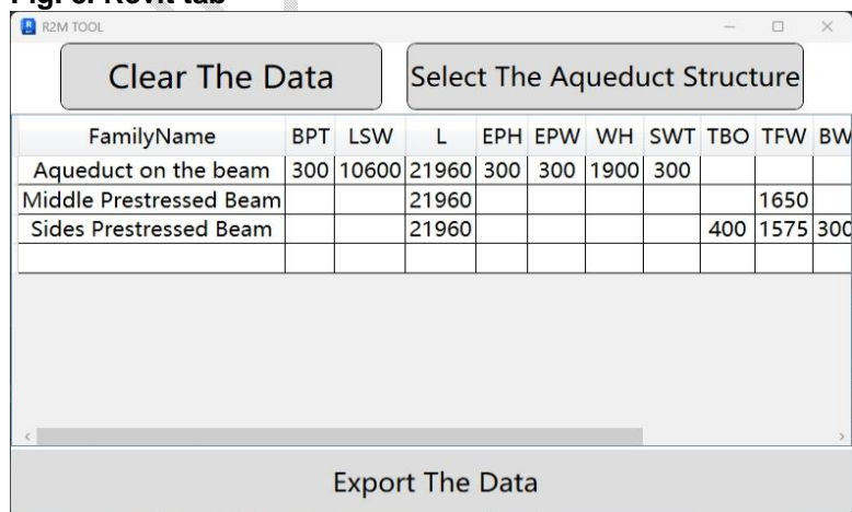
Fig. 5. Revit tab
