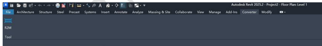
Fig. 5. Revit tab
