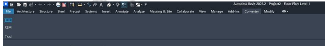
Fig. 5. Revit tab
