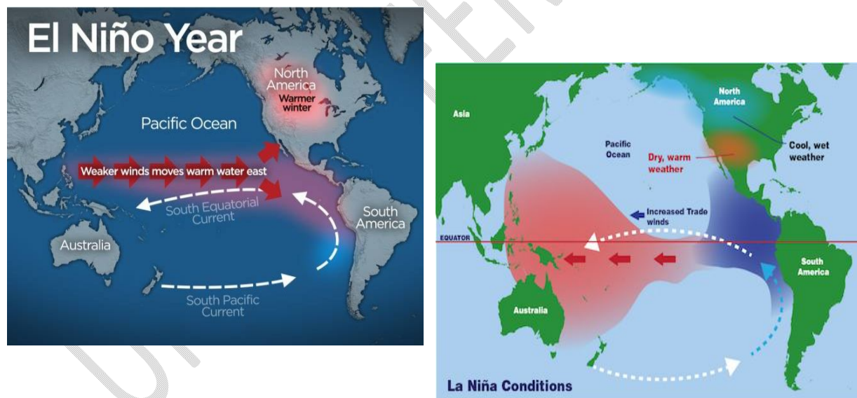
Fig. 1: a) El Niño b) La Niña
