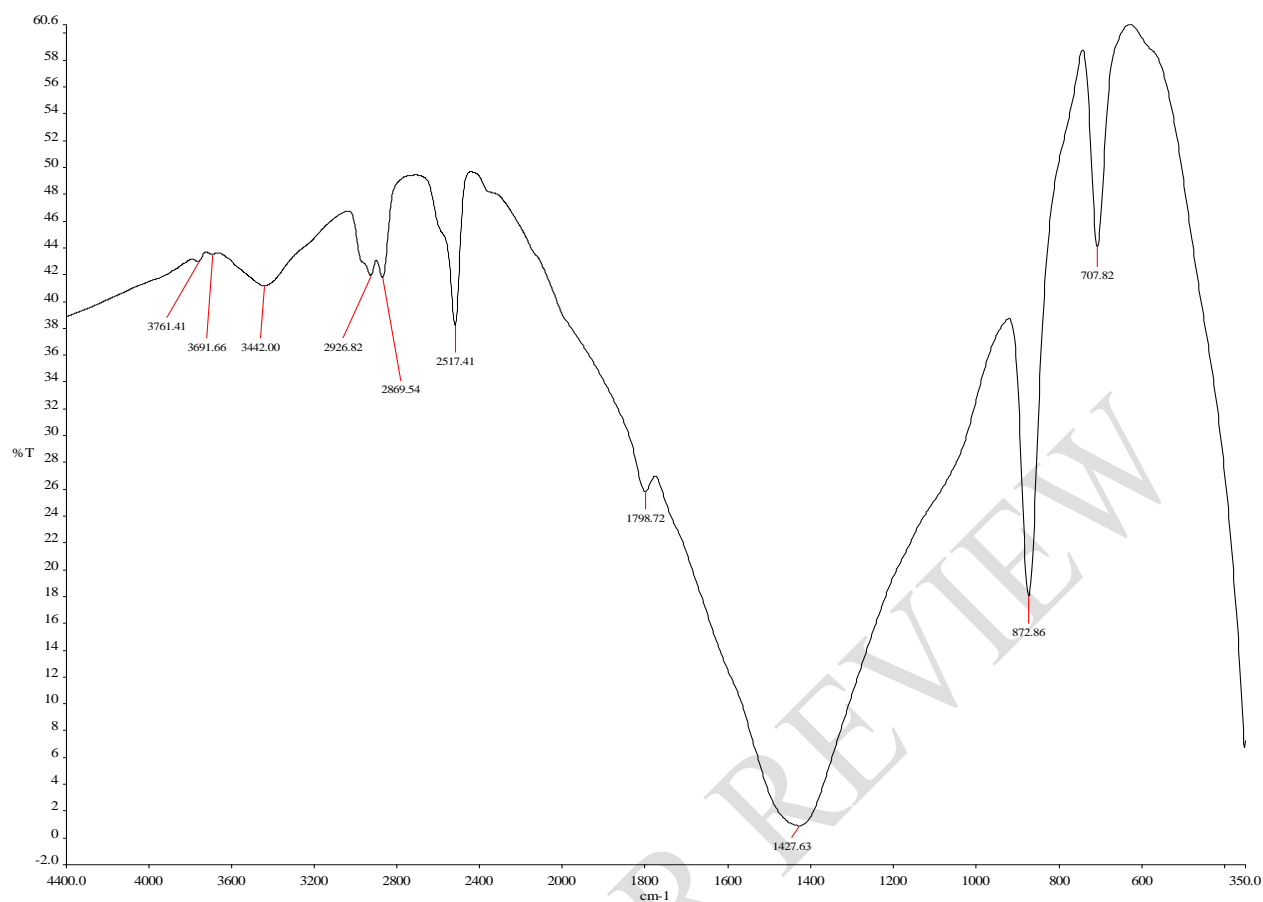
Fig11. Eggshell Calcined at 600 °C (KA)
