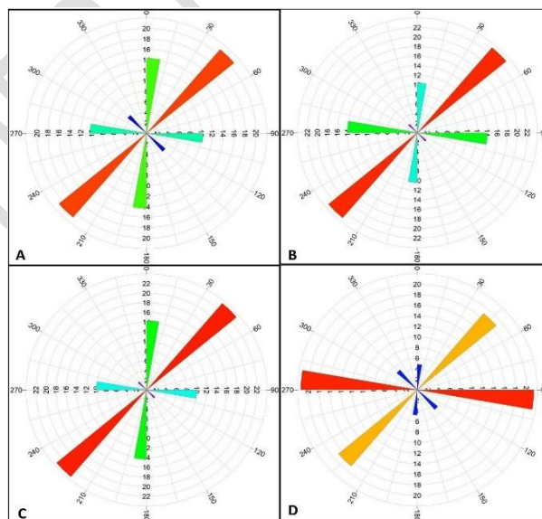
Figure7:Rosesdiagram.a.ASstructuresb.FVDstructuresc.HGMstructuresandd.CETstructuresfromRTE
