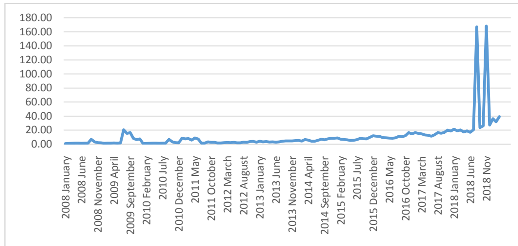
Fig. 2. Web Transactions
