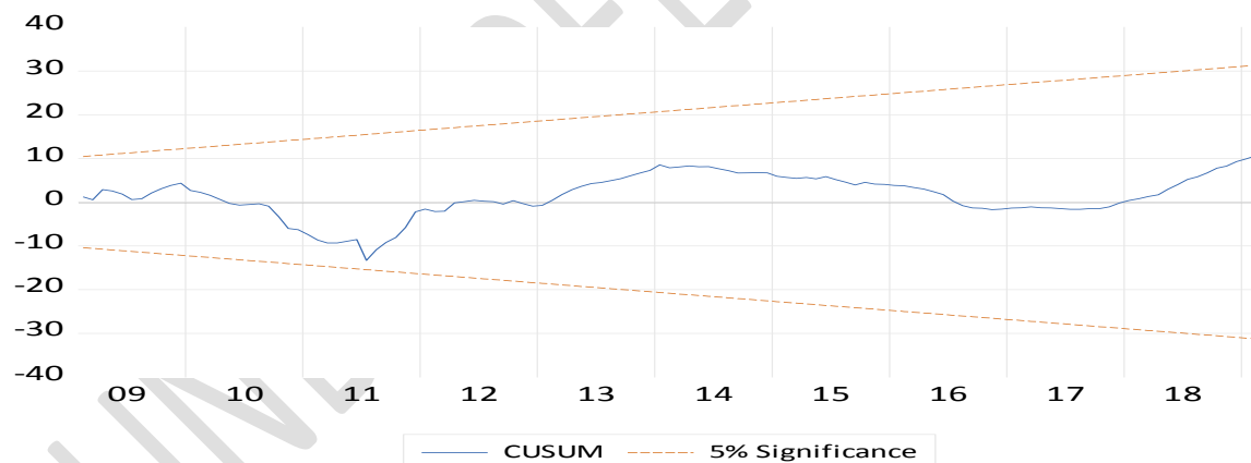
Fig. 6. CUSUM TEST
