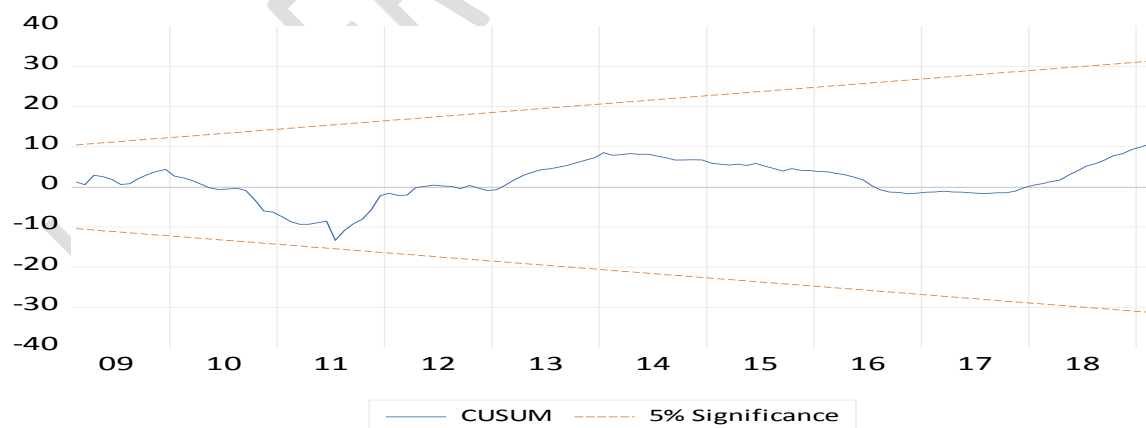
Fig. 6. CUSUM TEST
