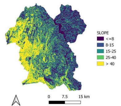
Fig. 7. Slope Map
