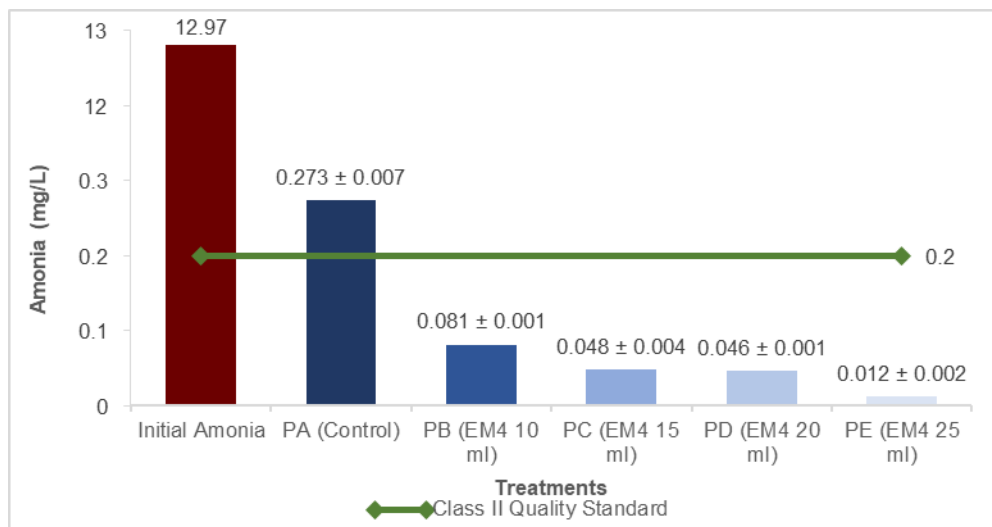
Fig 3. Ammonia Value
