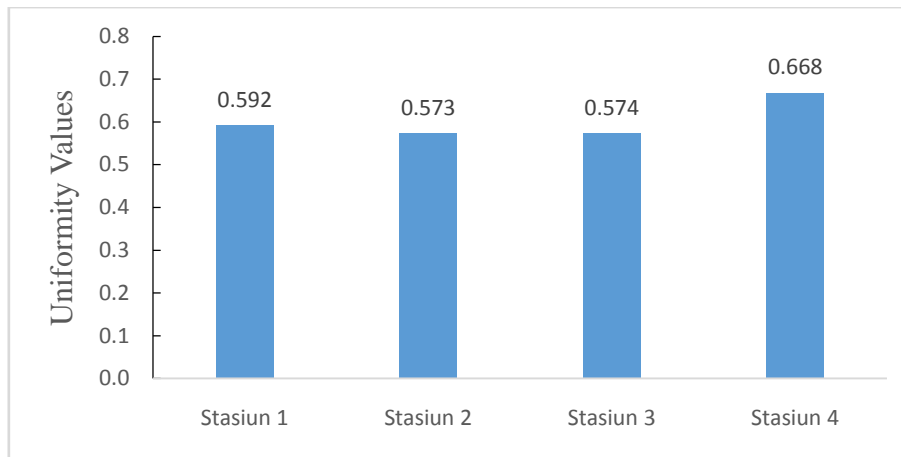
Fig 11. Macrozoobenthos uniformity values
