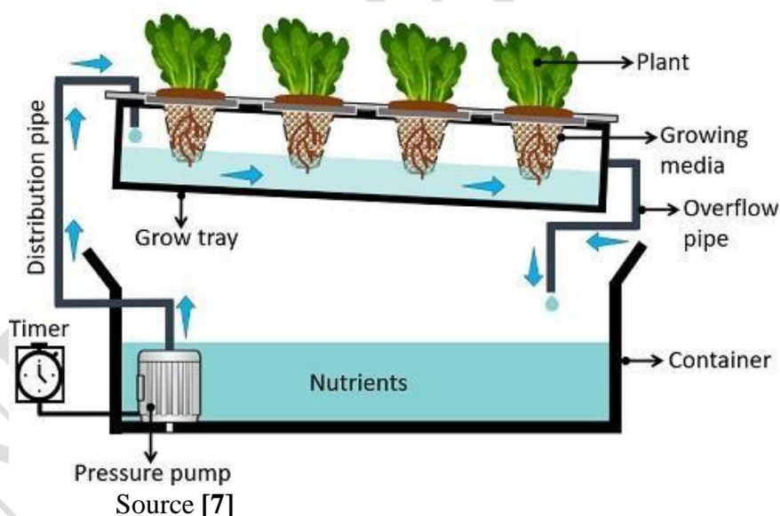
Fig 2. Nutrient film technique.
