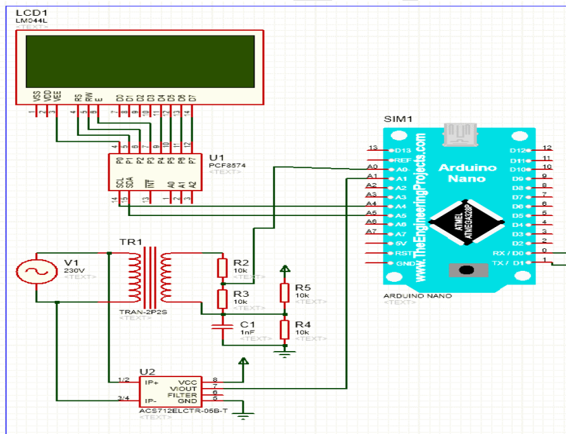
Fig. 6. Display Unit
